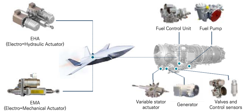
무인기용 작동기 및 엔진 보기류 (Actuators and engine accessory parts for UAV)
