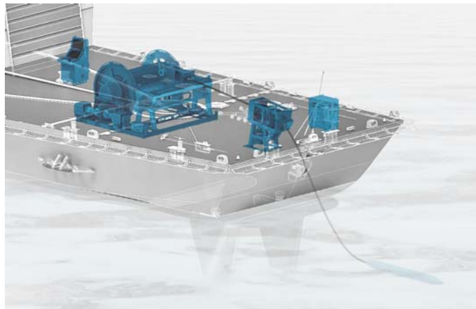
유압식 원치 시스템 | 전기식 원치 시스템 | 전원공급장치, 제어기
