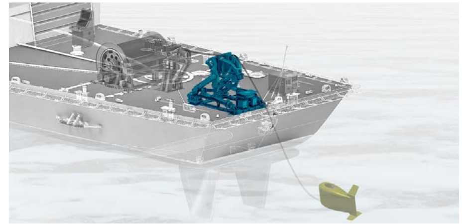
링크구조물 | 메인 실린더 | 그리퍼조립체 | 서브 실린더
